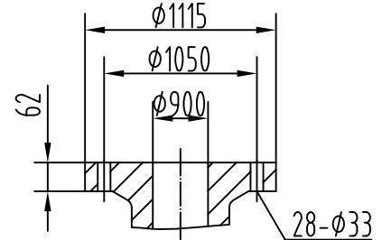
Outlet Flange (1.0Mpa)
