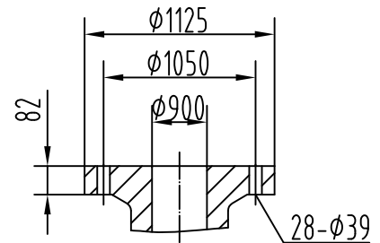
Outlet Flange (1.6Mpa)
