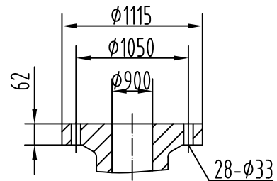
Outlet Flange (1.0Mpa)
