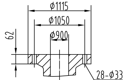
Outlet Flange (1.0Mpa)
