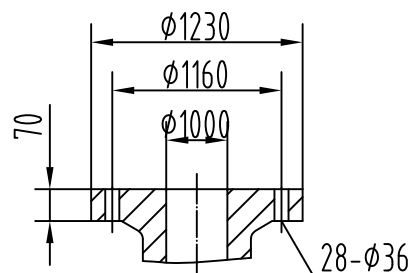
Outlet Flange (1.0Mpa)
